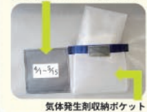
気体発生剤収納ポケット
